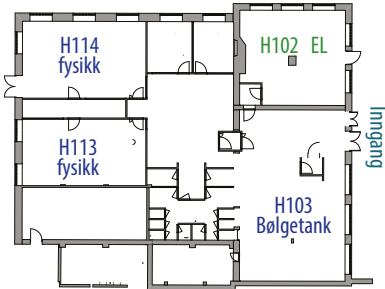
1. ETASJE
